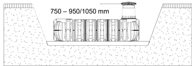
Trinkwasser-Teleskop-Domschacht
